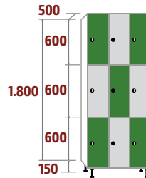
FMP-30/3 COD: 53539 89kg · 0,80m 3
