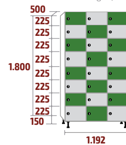
FZP-40/3 COD: 53626 159kg · 1,07m 3
