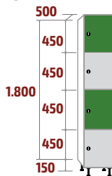
FCP-30/1 COD: 53521 37kg · 0,28m 3
