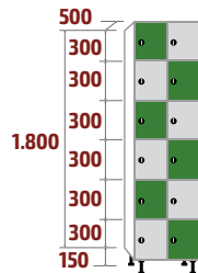
FBP-30/2 COD: 53562 78kg · 0,54m 3
