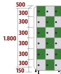
FBP-30/3 COD: 53569 113kg · 0,80m 3
