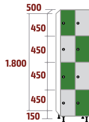
FCP-30/2 COD: 53522 67kg · 0,54m 3
