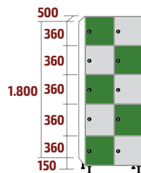
FPP-40/2 COD: 53566 88kg · 0,72m 3
