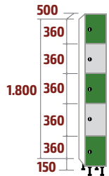
FPP-30/1 COD: 53551 40kg · 0,28m 3
