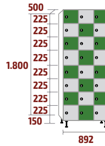
FZP-30/3 COD: 53589 129kg · 0,80m 3
