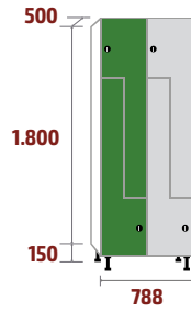
FLP-40/2 COD: 53546 80kg · 0,71m 3
