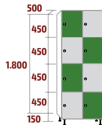
FCP-40/2 COD: 53526 81kg · 0,72m 3
