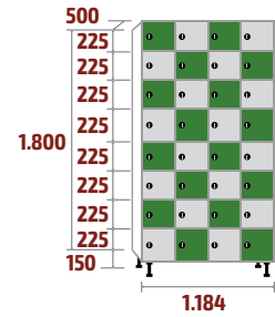
FZP-30/4 COD: 53625 170kg · 1,07m 3
