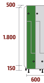
FLP-30/2 COD: 53542 70kg · 0,54m 3
