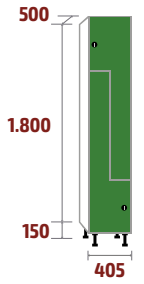
FLP-40/1 COD: 53545 44kg · 0,36m 3
