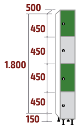
FCP-30/1 COD: 53521 37kg · 0,28m 3
