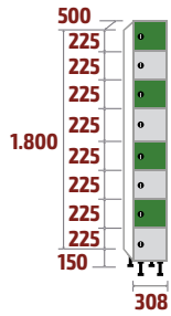
FZP-30/1 COD: 53581 48kg · 0,28m 3
