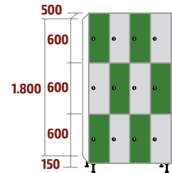
FMP-30/4 COD: 53609 116kg · 1,07m 3
