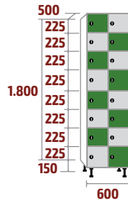
FZP-30/2 COD: 53582 89kg · 0,54m 3
