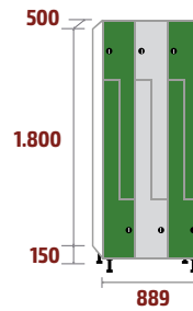
FLP-30/3 COD: 53549 101kg · 0,80m 3
