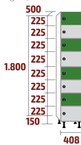
FZP-40/1 COD: 53585 57kg · 0,37m 3
