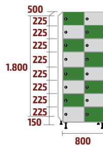
FZP-40/2 COD: 53586 108kg · 0,72m 3
