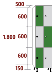
FMP-30/2 COD: 53532 62kg · 0,54m 3
